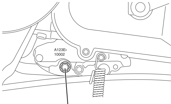
ドレンボルト \times 23Nm(2.3kgf·m)
