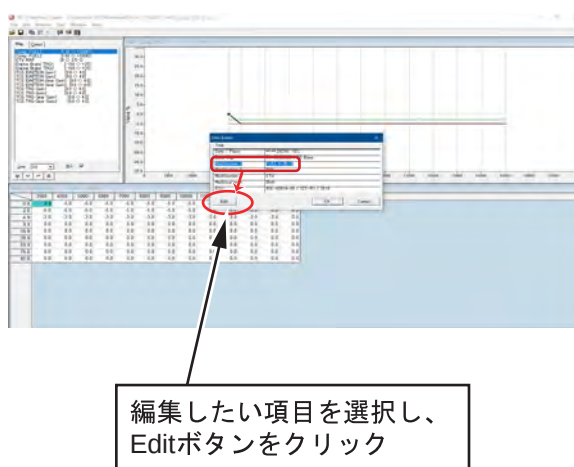
図 21：Title Editor ダイアログ
