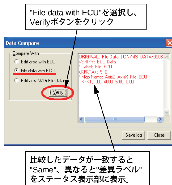
図 28 : Data Compare ダイアログ (File data with ECU)
