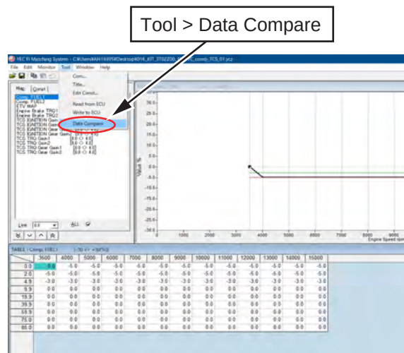
図 26：Data Compare ダイアログ起動
