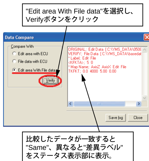
図 29 : Data Compare ダイアログ (Edit area with File data)
