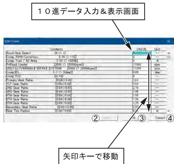
図 43：Edit Const ダイアログ
