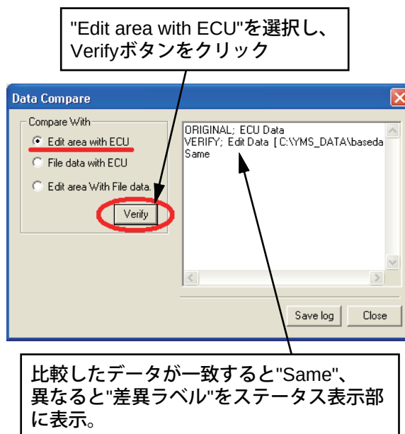
図 27： Data Compare ダイアログ（Edit area with ECU）
