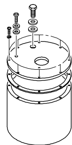
インナーハル (IH01) TD28 仕様
