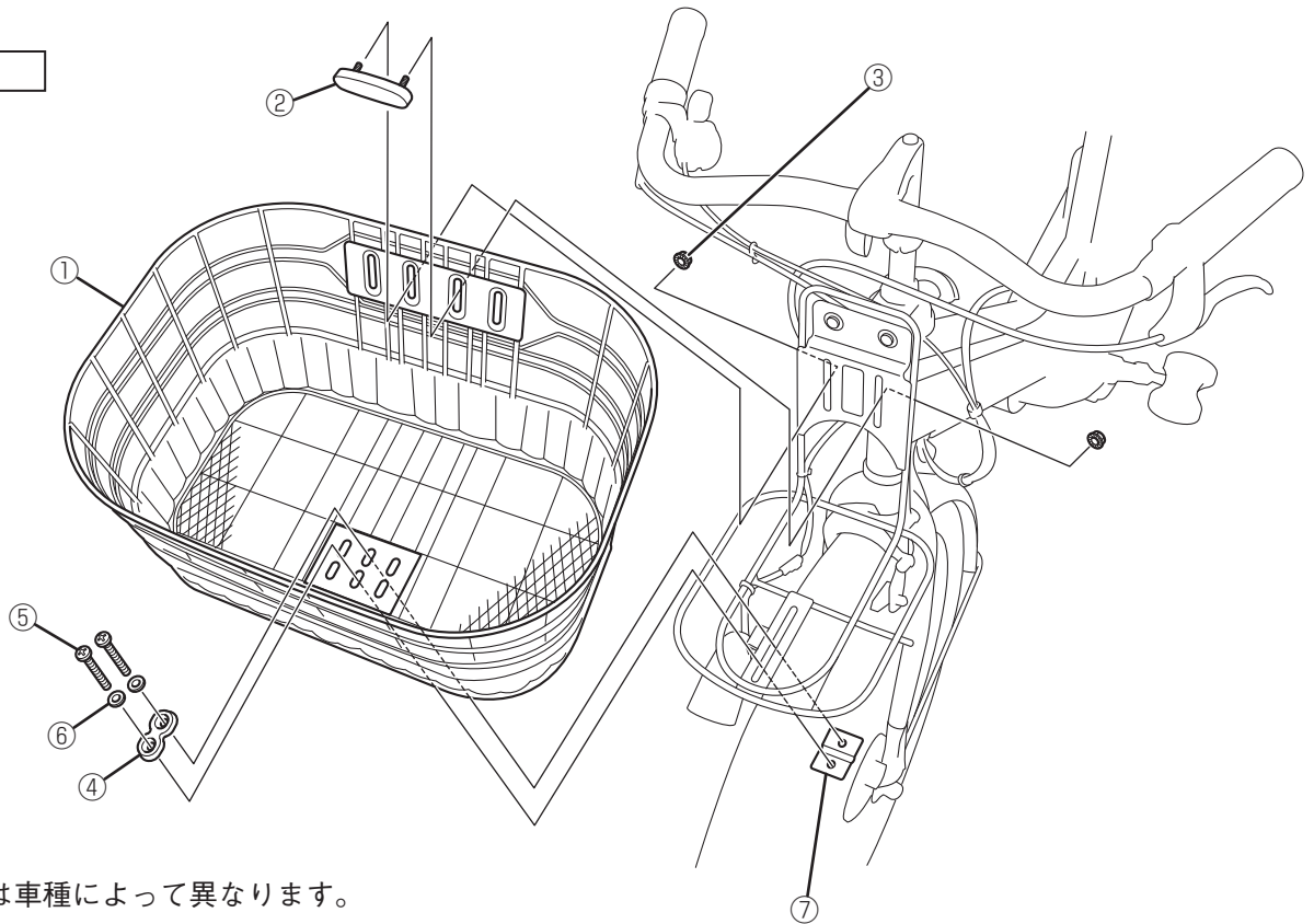
取付例
