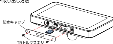
microSDカードスロット USB Type-Cポート ※USB-Type-Cポートはデータ通信用です(本製品では使用しません)。 給電用ではありませんのでモバイルバッテリーなどは接続しないでください。
