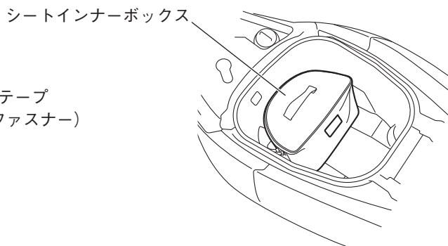
取付例
