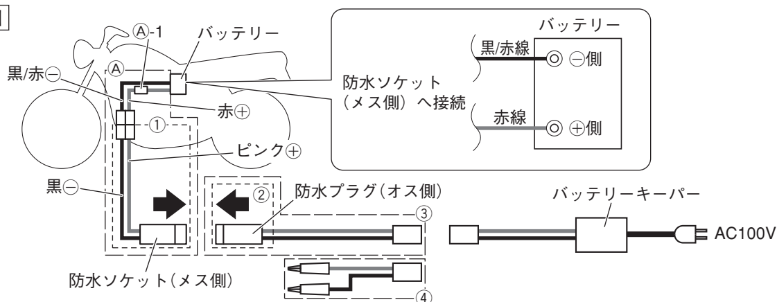
配線参考図
