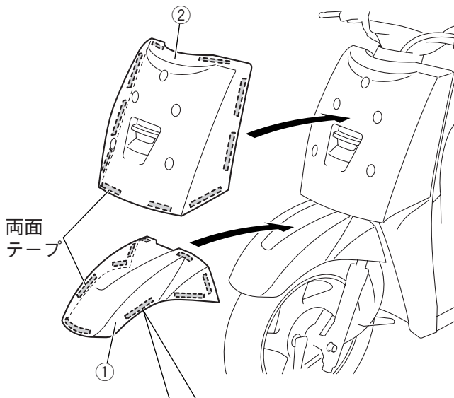
フロントフェンダ①、レッグシールド②貼り付け位置
